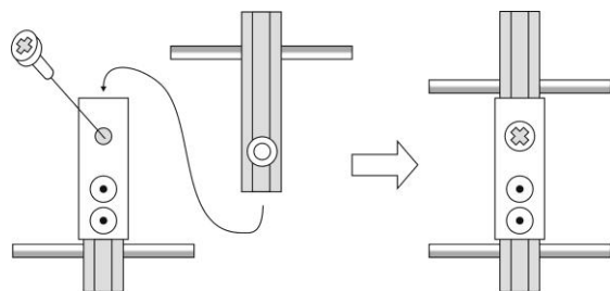
Рисунок 2. Сборка антенны.
