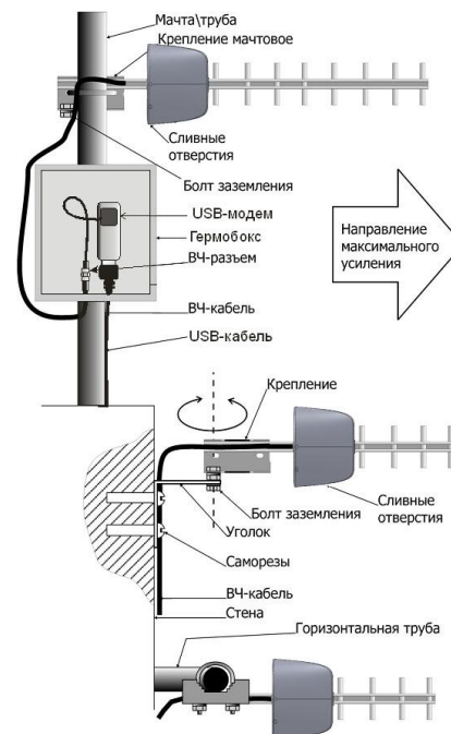
Рисунок 2 – Крепление антенны
